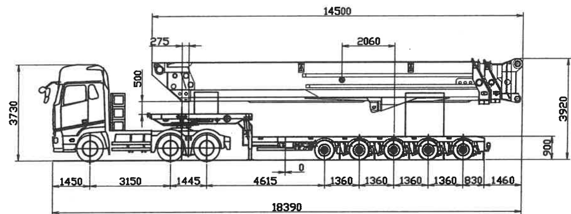
伸縮5軸 550t メインブーム運搬荷姿図 S=1/80
