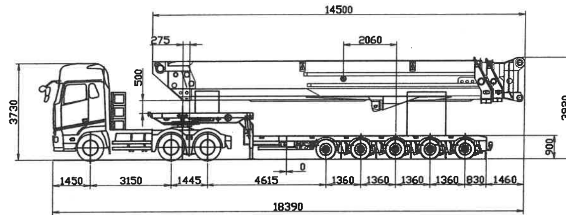
伸縮5軸 550t メインブーム運搬荷姿図 S=1/80
